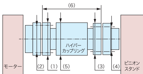
A.モーター～ピニオンスタンド間に設置の場合
