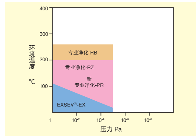
图 3-3 适用于净化度 100 的 EXSEV 轴承
