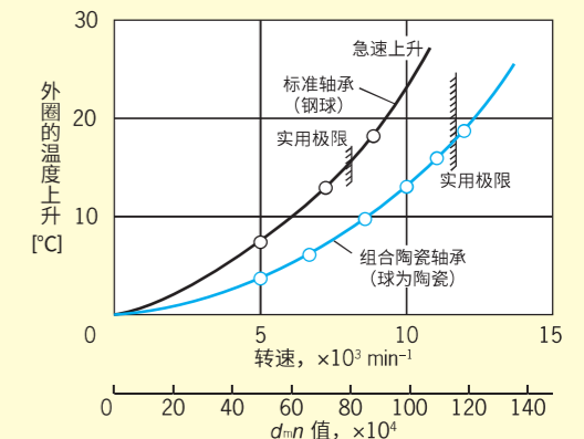
图 3 组合陶瓷轴承和标准轴承的升温特性比较
