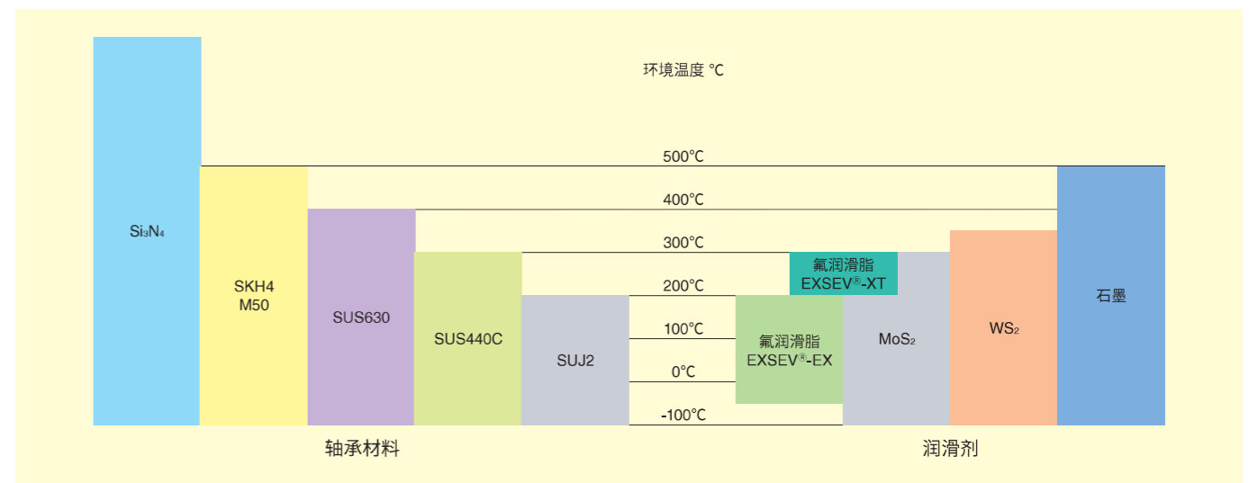
图 3-5 高温用的轴承材料和润滑剂
