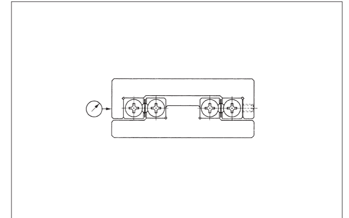
图 5-10 预紧调整方法示例
