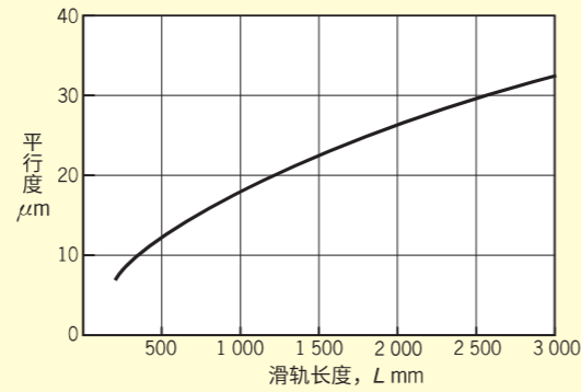
图 5-2 直线导轨 (类型 2) 行走时的平行度
