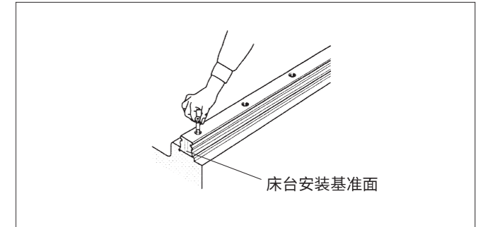
图 5-4 滑轨的半固定
