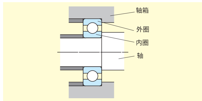
图 1-11 轴承的配合
