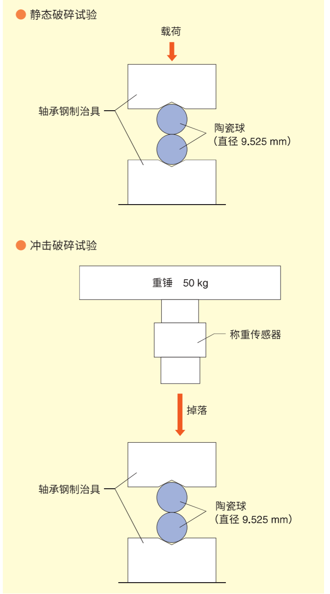
图 1-10 陶瓷球的破碎试验方法
