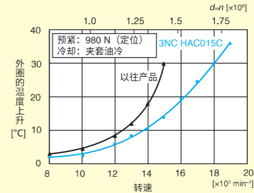
使用陶瓷球的轴承相互比较 (轴承尺寸: φ75×φ115×20mm)
