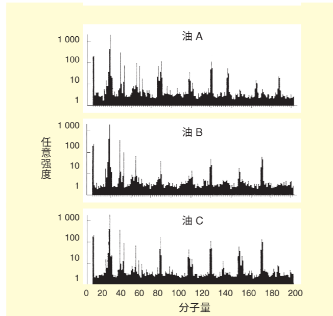
图 2-1 PFPE 的真空中释放气体比较
