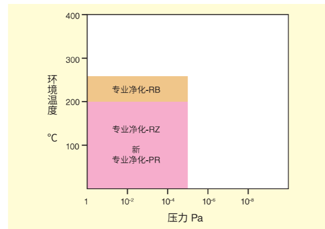
图 3-4 适用于净化度 10 的 EXSEV 轴承
