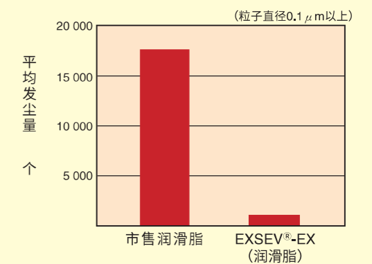
用于滚动轴承时的发尘特性 (每 2.83×10 -3 m 3 (0.1ft 3 ) 的个数)
