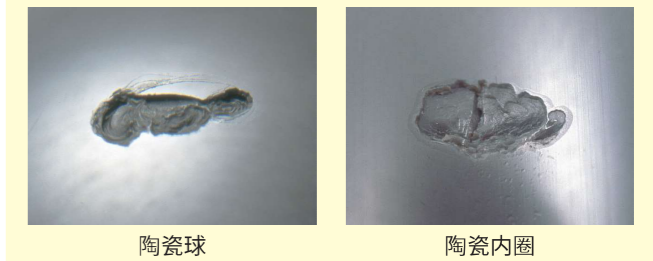
图 1-5 陶瓷上出现的剥离
