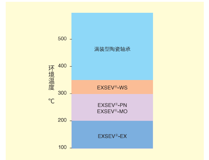
图 3-6 适用于高温的 EXSEV 轴承
