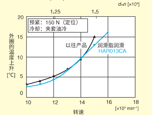
图 2 变更为润滑脂润滑后的高速性能比较
