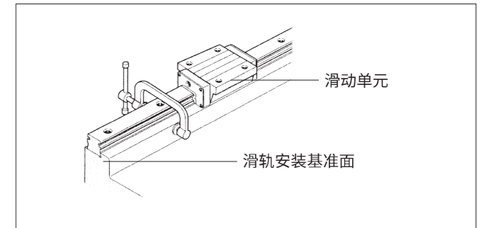
图 5-5 基准侧滑轨的固定
