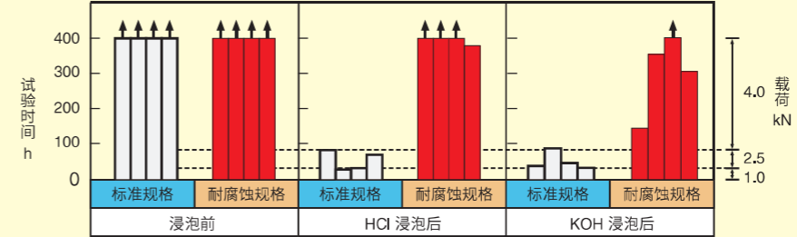
浸泡到酸、碱溶液后的寿命比较
