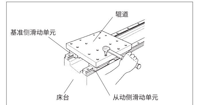
图 5-6 滑动单元的固定
