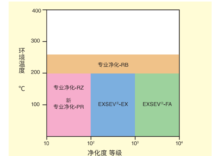
图 3-1 适用于净化环境的 EXSEV 轴承
