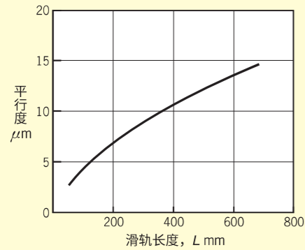
图 5-1 直线导轨 (类型 1) 行走时的平行度
